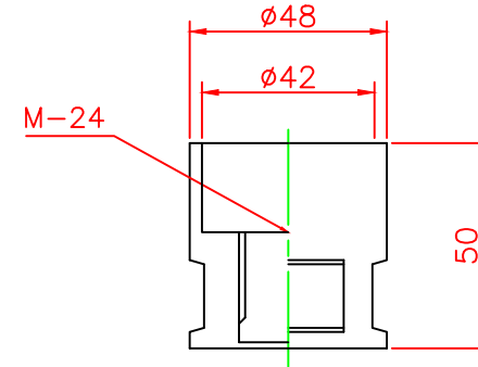
アンカー部形状図
